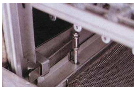
Os tubos de descarga com comando estão localizados acima do nível do filtro e estão interligados com as portas
