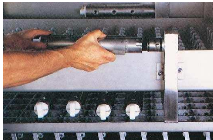
Braços de lavagem com juntas de ligação rápida
