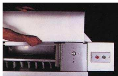
Painel de saída desmontável para facilitar a inspecção e a limpeza
